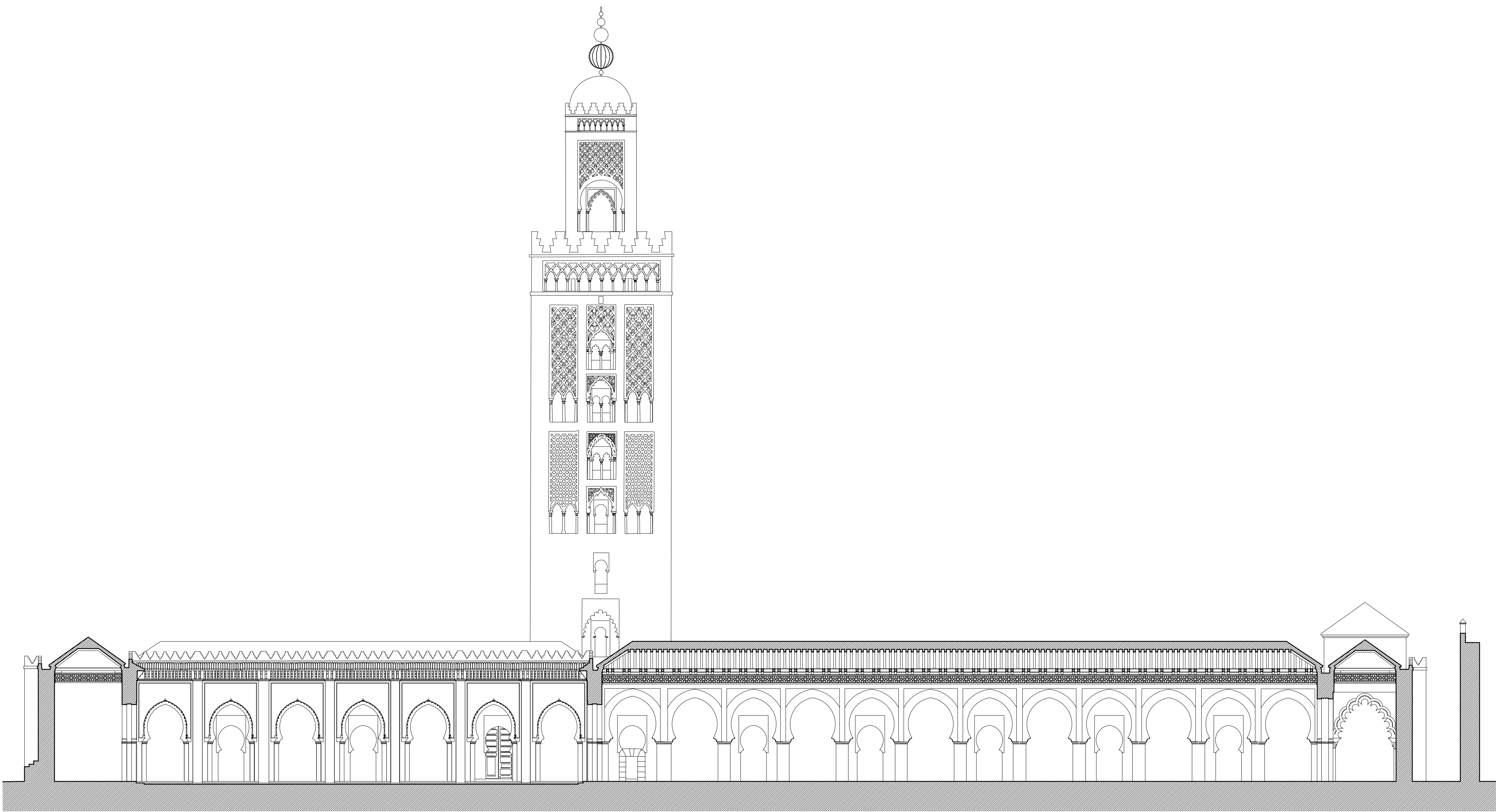
MEZQUITA ALMOHADE DE SEVILLA. SECCION LONGITUDINAL.
