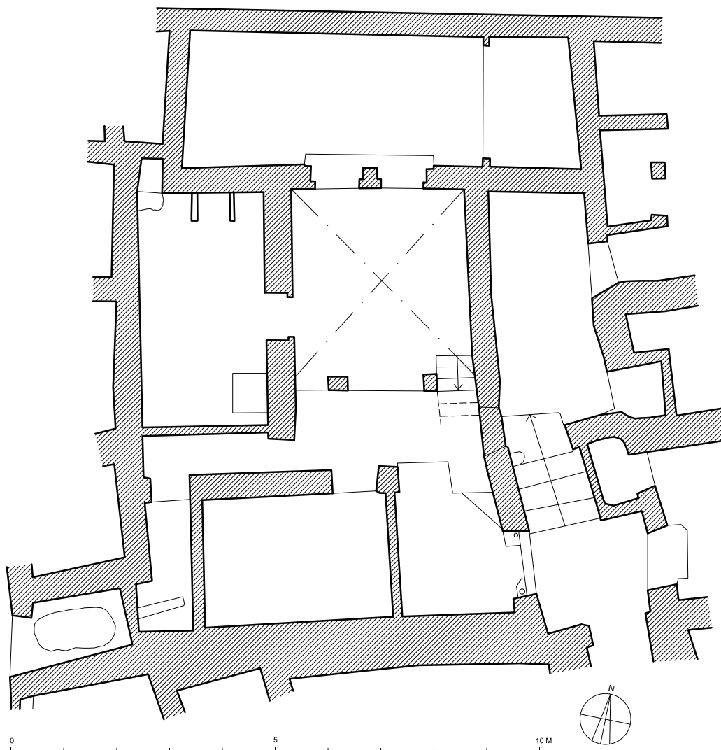
SIYASA (CIEZA, MURCIA) CASA nº 10. PLANTA Basado en planimetría de J. Navarro
